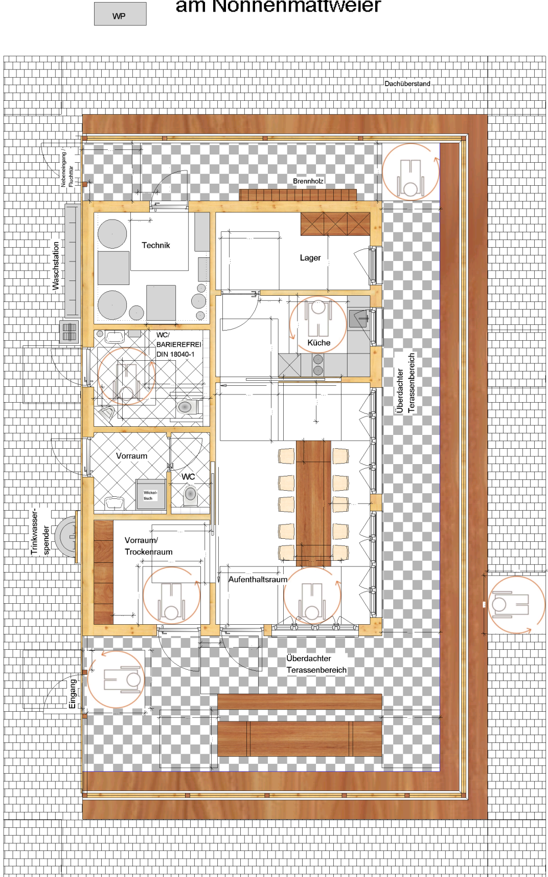
Grundriss der "Barrierefreien" Schutzhütte "Zur Blauen Stunde" am Nonnenmattweier
